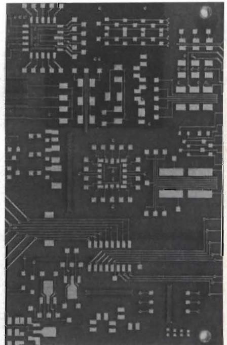
Tipiche strutture del rame dei circuiti stampati utilizzati per il montaggio dei componenti SMD.
