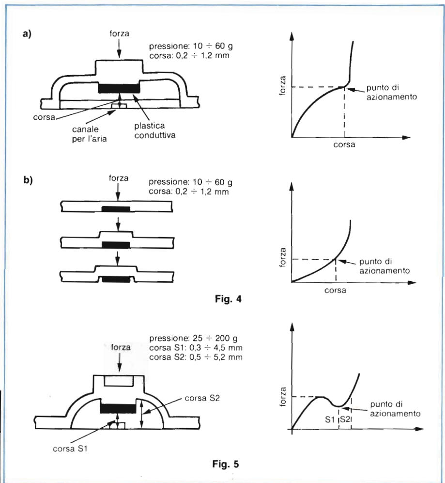
Fig. 4 - Tastiere senza risposta tattile, a pareti verticali (a) e di tipo completamente piatto (b).
