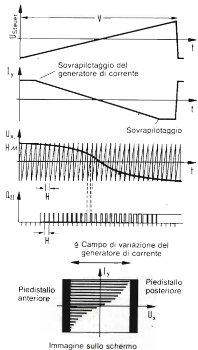
Fig. 3. Diagramma dell'elaborazione del segnale per la produzione del grafico a colonne.
