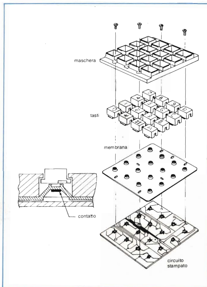
Fig. 1 - La vista esplosa mostra la semplicità costruttiva della tastiera a membrana.
