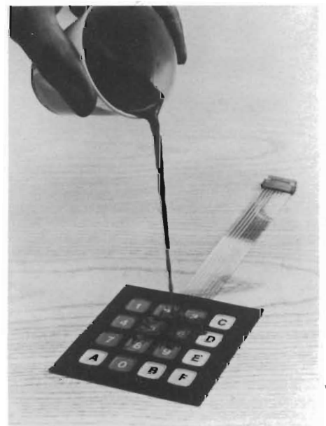
Fig. 2 - Tastiera a membrana, TC 31, Micro Switch, con tasti numerici (3 x 3) od alfanumerici (4 x 4). I colori, la grafica e i formati sono forniti secondo le specifiche del cliente. La fotografia indica come queste tastiere siano completamente protette dagli agenti esterni. La parte posteriore autoadesiva permette una facile ed economica installazione.
