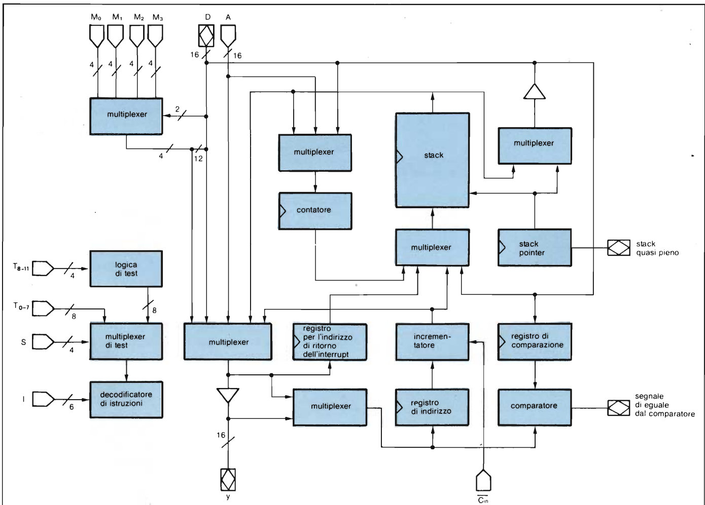
Fig. 3 - Il sequenziatore Am29331, micro-interruibile.
