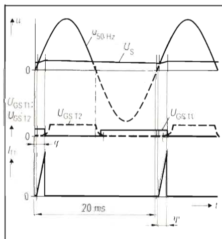
Fig. 2 - Andamento delle tensioni e delle correnti nel circuito di fig. 1.
