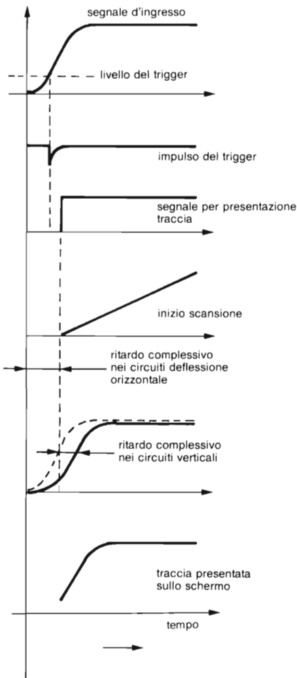
Fig. 9 - A causa dei ritardi introdotti sia dal circuito di trigger che da quello di scansione, la porzione iniziale di un segnale non potrebbe apparire sullo schermo del CRT di un oscilloscopio. Questo inconveniente viene eliminato inserendo una linea di ritardo nel canale di amplificazione verticale (canale del segnale). In alto, è indicato il segnale che si vuole osservare, in basso, come apparirebbe in realtà questo segnale sul CRT se non ci fosse la linea di ritardo; al centro, posizione del segnale di scansione rispetto al segnale che si vuole osservare.
