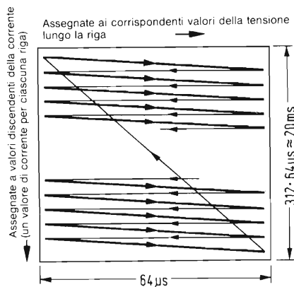
Fig. 1. Schema del processo di formazione di un'immagine televisiva. Esso costituisce la base del funzionamento del tracciatore di curve caratteristiche video.
