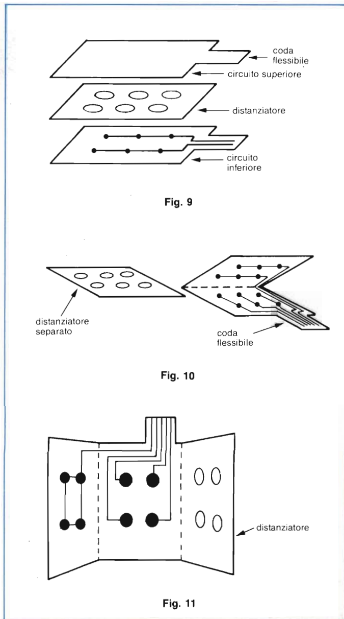
Fig. 11 - Un solo foglio costituisce tutti e tre gli elementi nel tipo a doppia piegatura.
