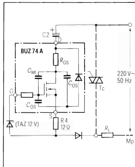
Fig. 5 - Sistema di protezione del transistor di potenza BUZ74A. Tra massa del circuito e il gate viene inserito un diodo soppressore veloce TAZ. Sono indicate anche le capacità interne del transistor.
