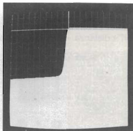
Fig. 19. Curva caratteristica IC - VCE di un transistor PNP BC178B, con IB = 30 μA. Scale: orizzontale 0,2 V/div. verticale 1 mA/div.
