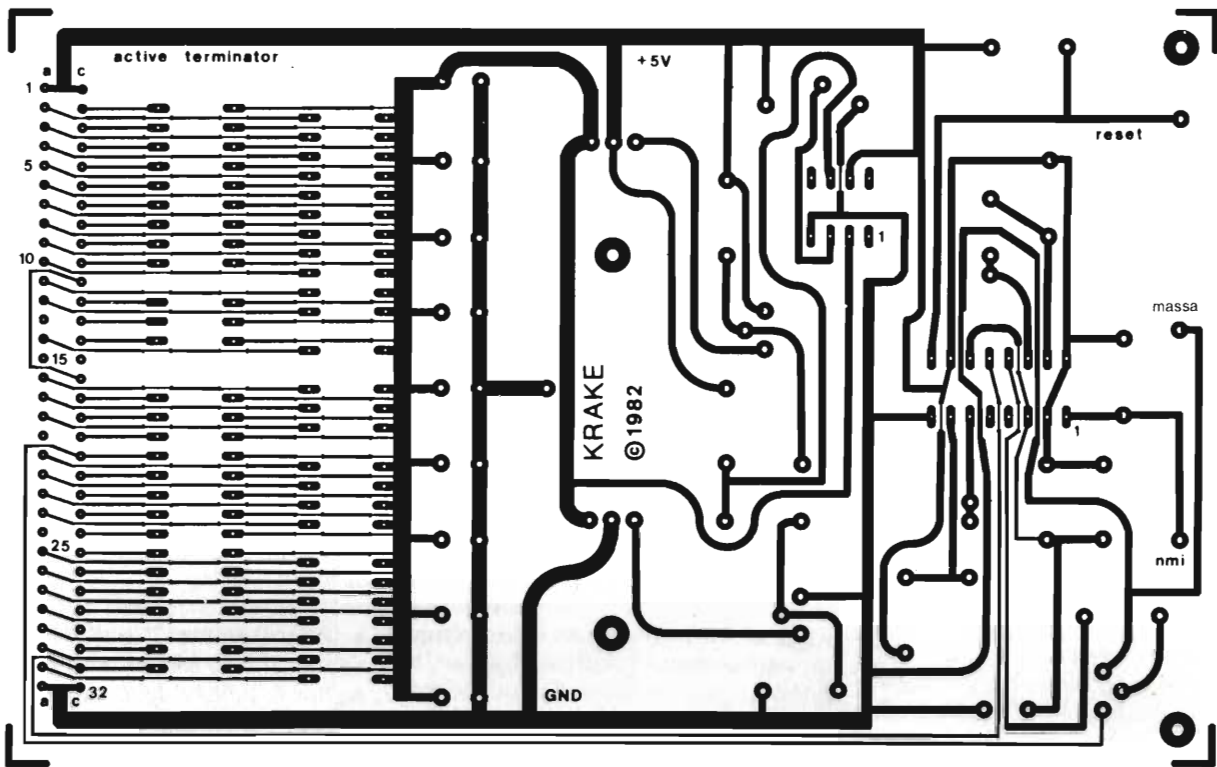
Fig. 4 - Layout della scheda formato Eurocard.
