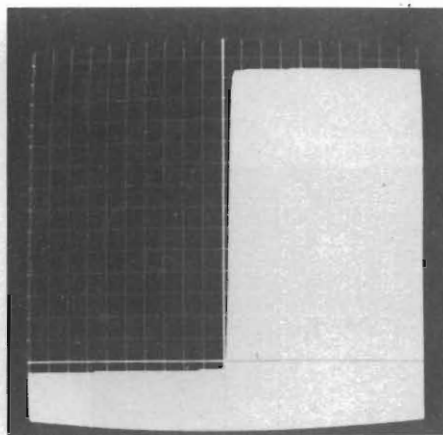
Fig. 18. Curva caratteristica IC - VCE di un transistor NPN 2N2218, con Ib = 30 μA. Scale: orizzontale 0,5 V/div. verticale 0,1 mA/div.
