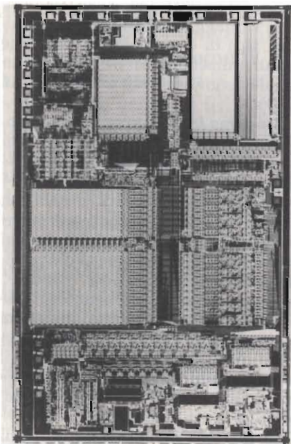
Fig. 2 - Struttura del chip del circuito integrato "Sicofi" (Signal-Processing Codec Filter). Contiene 36.000 transistori combinati in tecnologie parte analogiche e parte digitali. È il primo chip codec-filter con filtri digitali in tecnologia CMOS. È richiesto in ogni circuito d'ingresso di una postazione-utente. Qui effettua tra l'altro complicate funzioni di commutazione e la conversione analogica-digitale.
