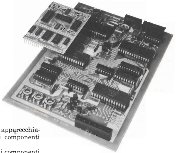
Fig. 2 - Due versioni di decodificatore per la ricezione di informazioni videotel: quello realizzato con componenti SMD, (in alto a sinistra) occupa un quarto della superficie di quello realizzato con normali componenti con terminali.
