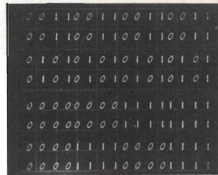
Fig. 2 - Come compaiono gli "uni" e gli "zeri" sullo schermo dell'oscilloscopio.
